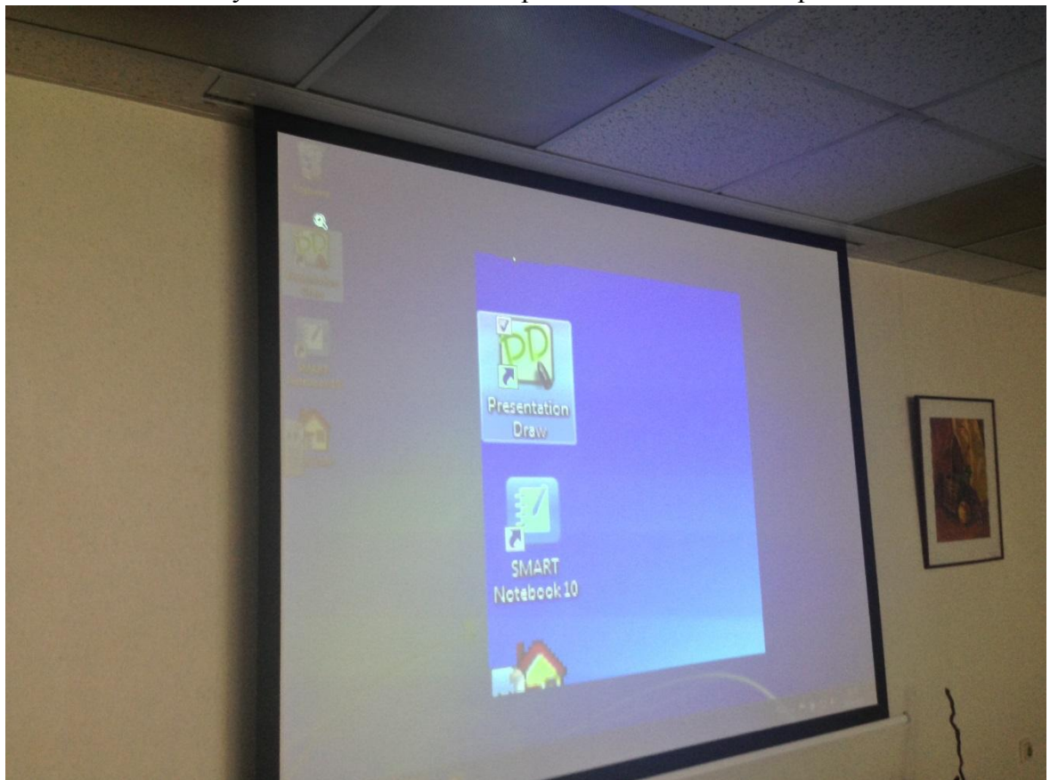
Рисунок 20. Увеличенное изображение.
