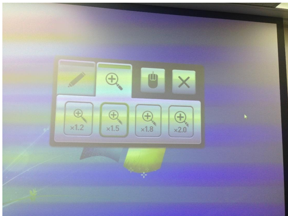
Рисунок 18. Функция Увеличение.
