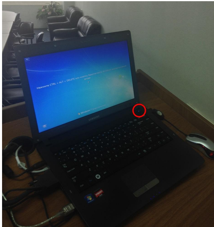
Рисунок 9. Включение компьютера.
